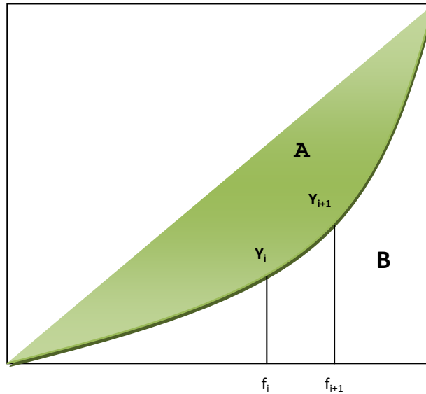
RAJAH 1/Figure 1 Keluk Lorenz/Lorenz Curve
